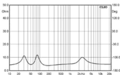
Sistema 30.50 - Impedenza
