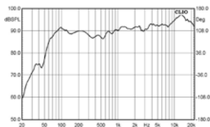
Sistema 30.50 - Risposta in frequenza
