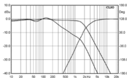
Sistema 30.50 - Risposta elettrica
